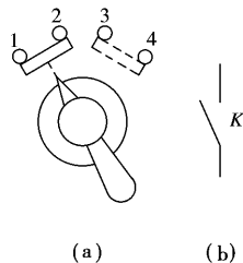
图 圆猿瑶主令开关结构示意图 (员)结构示意图 (圆)触头符号
