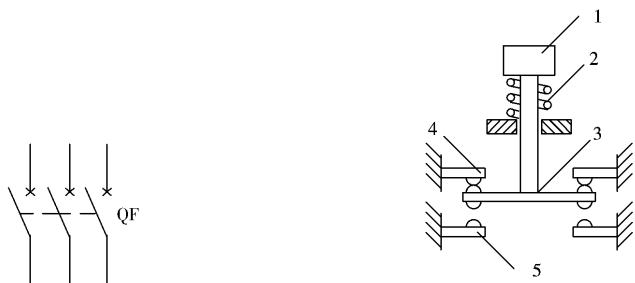
图 圆猿瑶自动开关符号图
