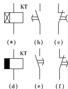
图 10-2 时间继电器符号
