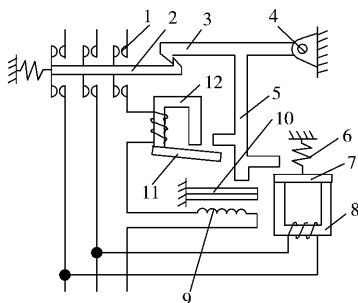
图 圆猿瑶自动开关结构原理图
