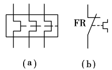
图 4-11 热继电器符号
