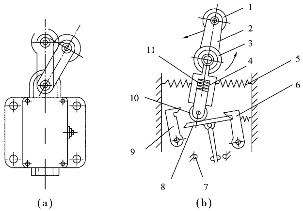
图 4-15 滚轮式行程开关 (a) 外形图 (b) 原理图
