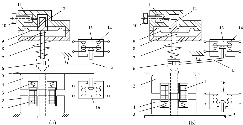
图 10-1 空气式时间继电器结构原理图
