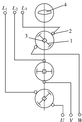
图 2-1 组合开关结构示意图
