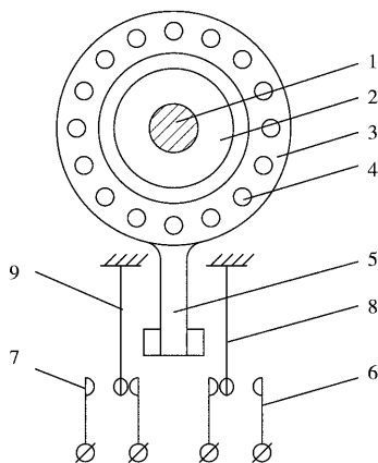
图 10-3 速度继电器原理示意图 1-转轴 2-转子 3-定子 4-绕组 5-摆锤 6-静触头 7-簧片 8-静触头 9-簧片
