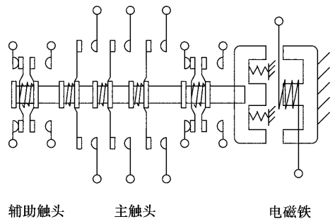
图 4-18 交流接触器结构原理图
