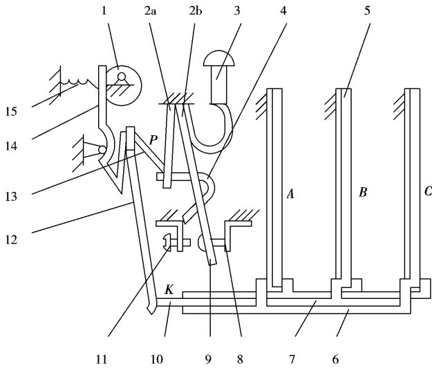
图 4-10 热继电器系列热继电器结构原理图
