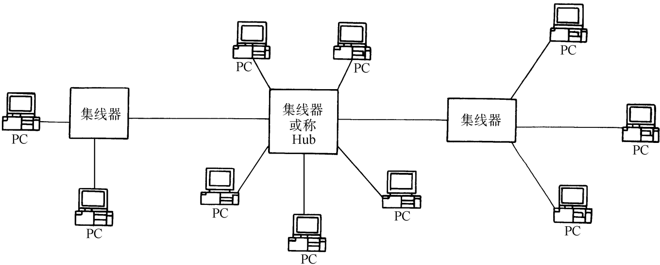
图 1-7 混合型拓扑
