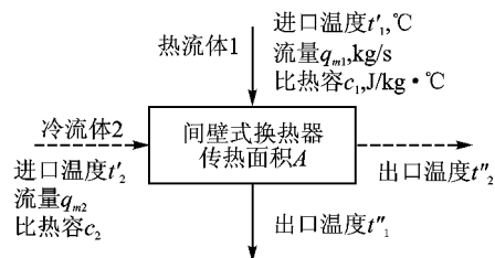
图 4-1 间壁式换热器的基本参数
