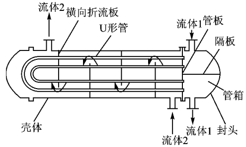
图 1-2 壳管式换热器
