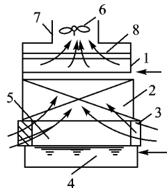
图 1-1 抽风逆流式水冷却塔示意图 1—配水系统 2—淋水装置; 3—百叶窗 4—集水池; 5—空气分配区 6—风机; 7—风筒 8—收水器
