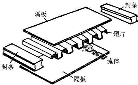
图 1-1 隔板翅式换热器的单元结构图
