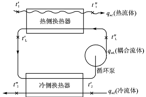
图 1-2 液体耦合间接式换热器
