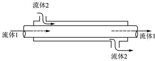
图 1-1 双套管式换热器
