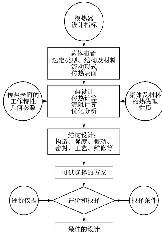
图 1-1 愿换热器设计过程框图
