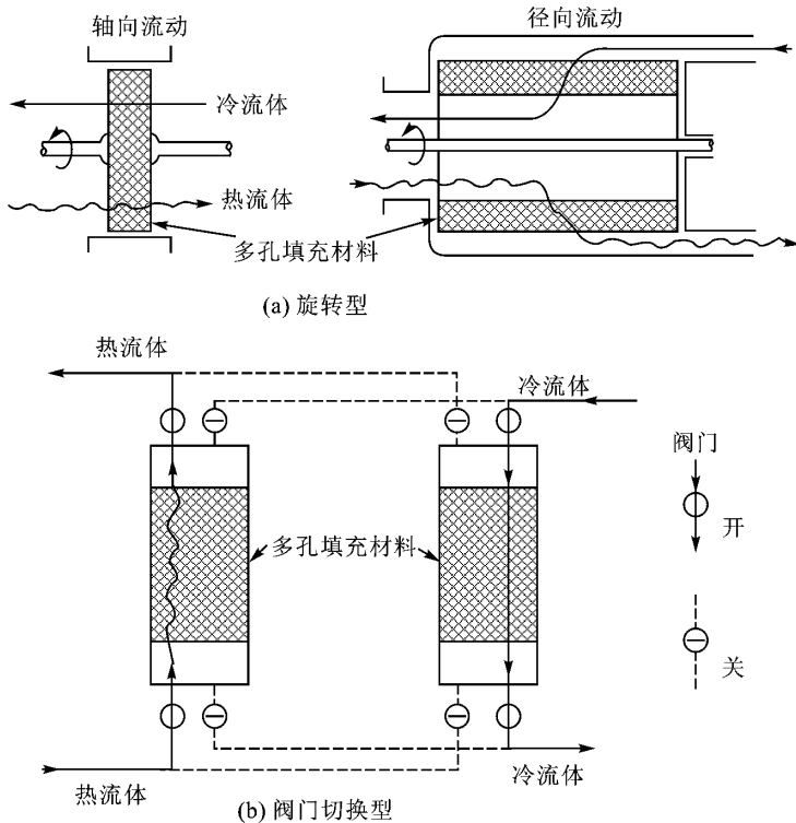
图 1-10 周期流动式换热器
