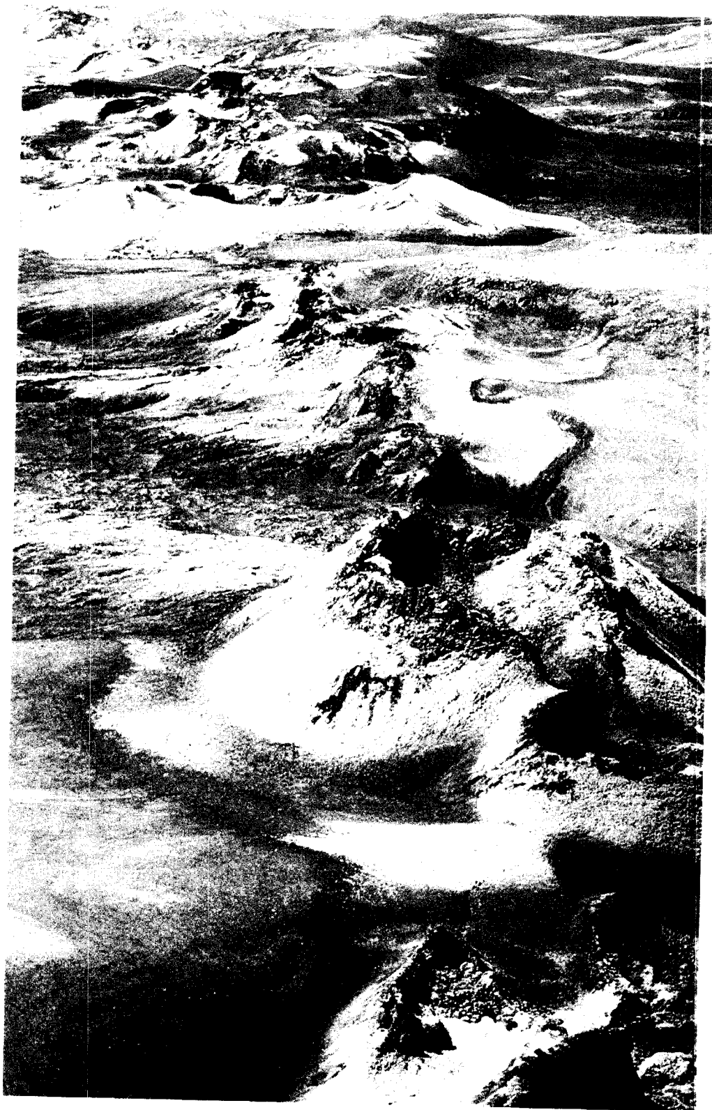
1-13 冰岛的斯凯弗塔裂谷，它是一道长27公里的裂谷的一部分，这个裂谷于公元1783年喷发，喷发出的大量火山灰和火山气体造成冰岛境内75%的动物死亡，并在之后的饥荒中更造成了一万多居民的死亡。人与其它动物的生命在自然的环境中还是相当脆弱的。
