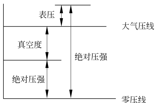
图 1-1 绝对压强、表压与真空度的关系
