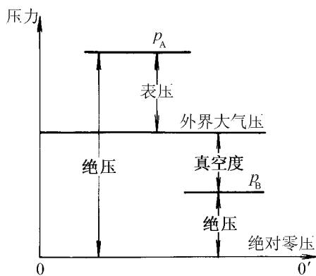
图 1.1-1 绝压、表压和真空度的关系
