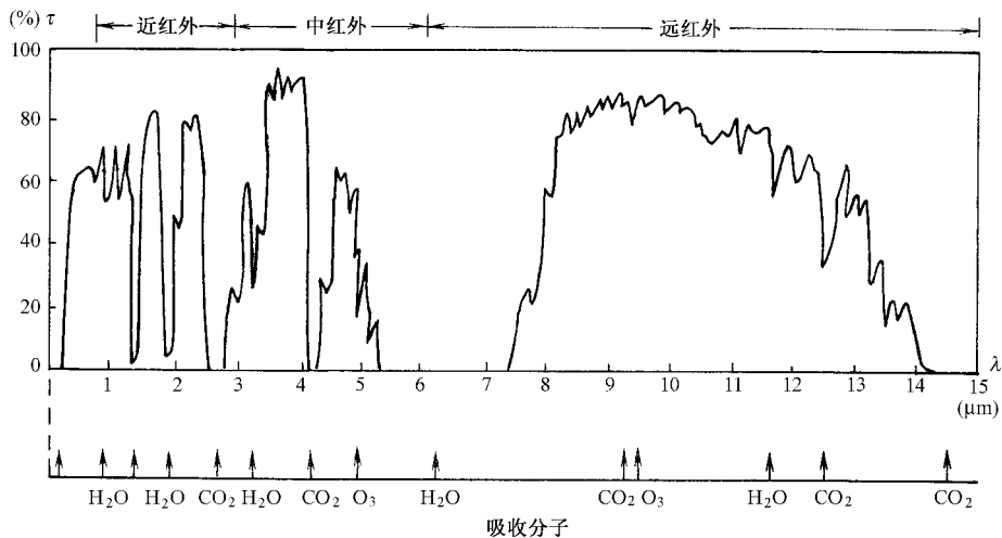
图 1-4 太阳光谱通过 1853m 长度的大气透射率曲线
