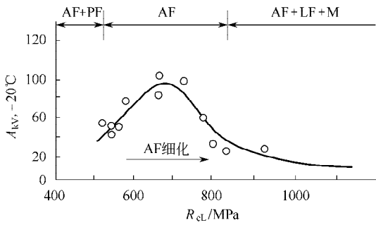
图 5-17 焊缝韧性与强度的关系
