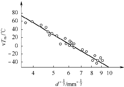
图 1-12 铁素体晶粒直径与 T_{18} 的关系 (断口中纤维区占线像)
