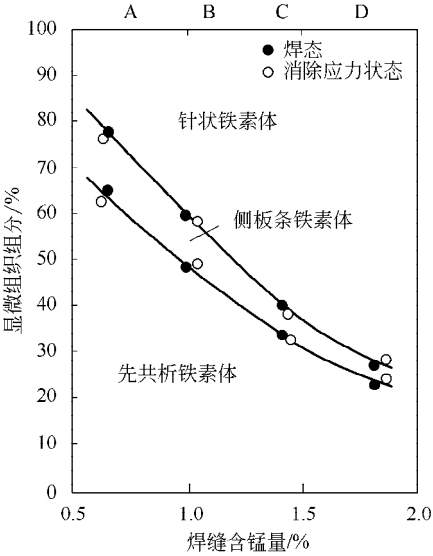
图 5-50 摇含锰量对盖面焊缝显微组织的影响
