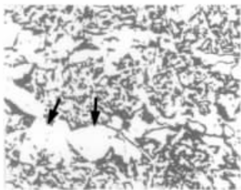
照片 晶界铁素体 伊原
