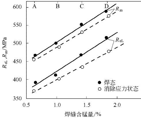
图 2 摇含锰量对焊缝拉伸性能的影响
