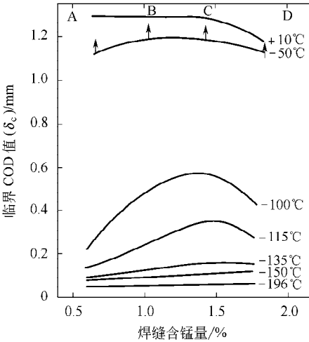
图 1-12 焊态下的 0.009% 值变化
