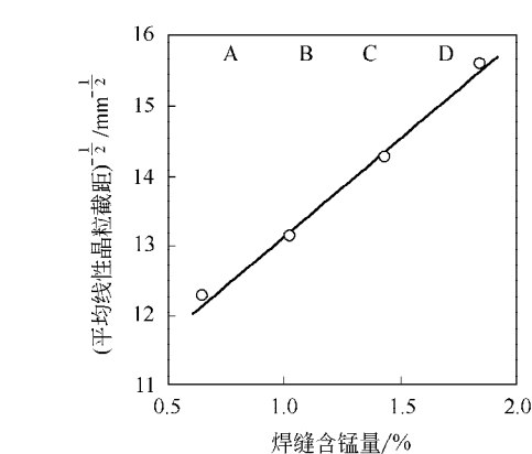
图 1 摇含锰量对细晶区晶粒线性截距的影响
