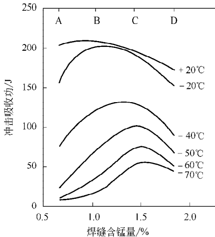
图 4 摇消除应力状态下的冲击吸收功变化
