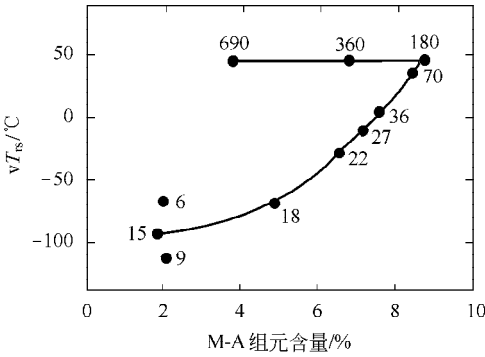
图 1-11 摇 Mn-A 组元数量对 \sigma_s 的影响 (图中数字为 \sigma_s ， \sigma_s 为 MPa)
