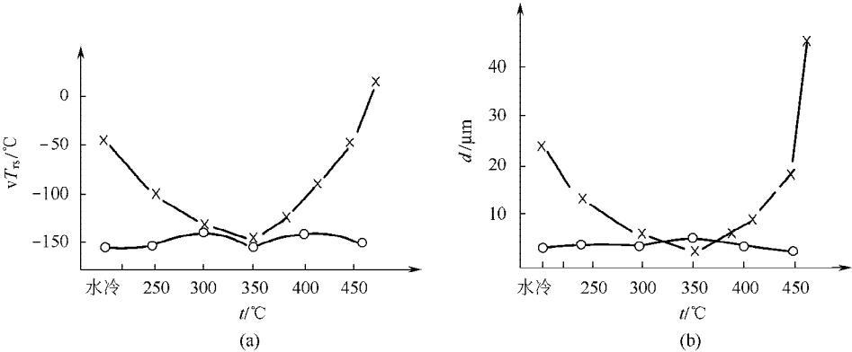
图 10-10 贝氏体形成温度对 增 与 图 的影响
