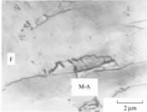
照片 1-11 淬硬组元 (伊文图)
