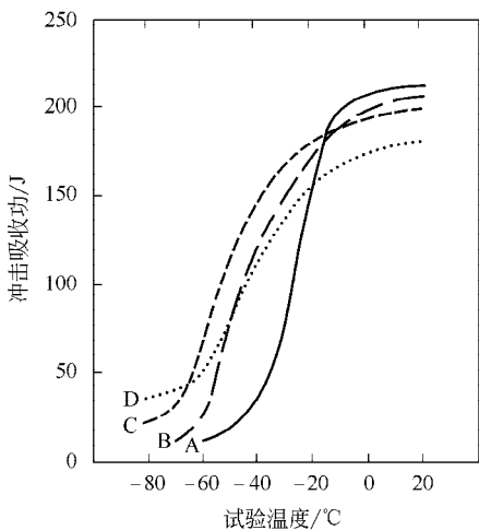
图 3 摇含锰量对焊态下冲击吸收功的影响
