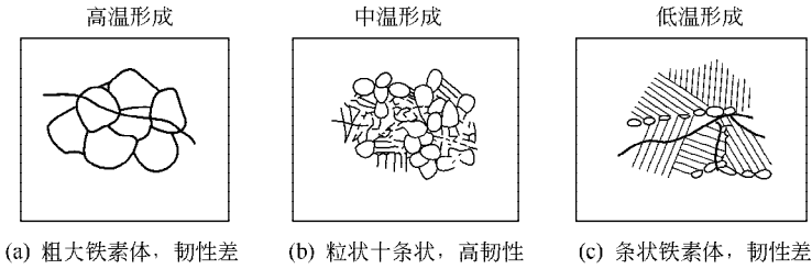
图 5-15 铁素体形貌及分布对韧性的影响
