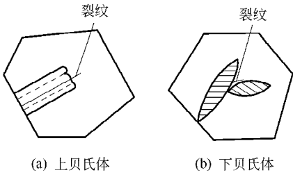
图 1-10 摇上贝氏体和下贝氏体抗裂纹扩展示意
