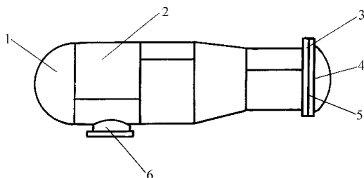
图 员圆 压力容器的简单构造
