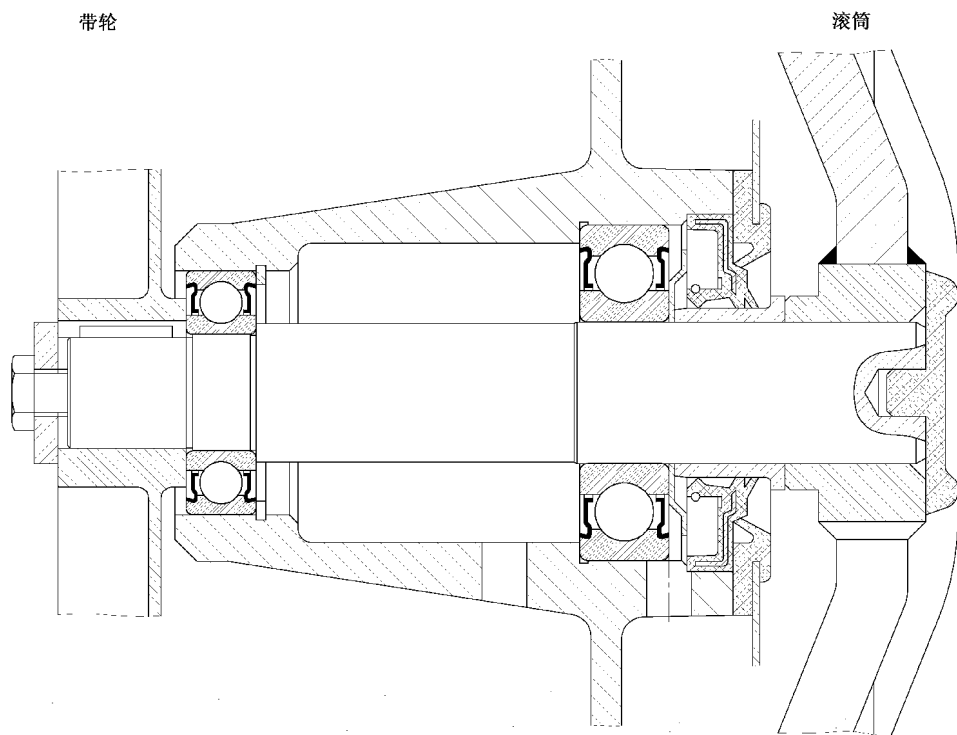
图 1-6 家用洗衣机滚筒装置
