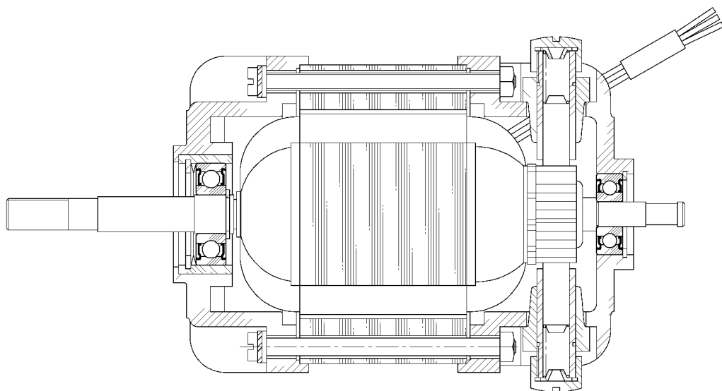
图 1-4 家用电器电动机
