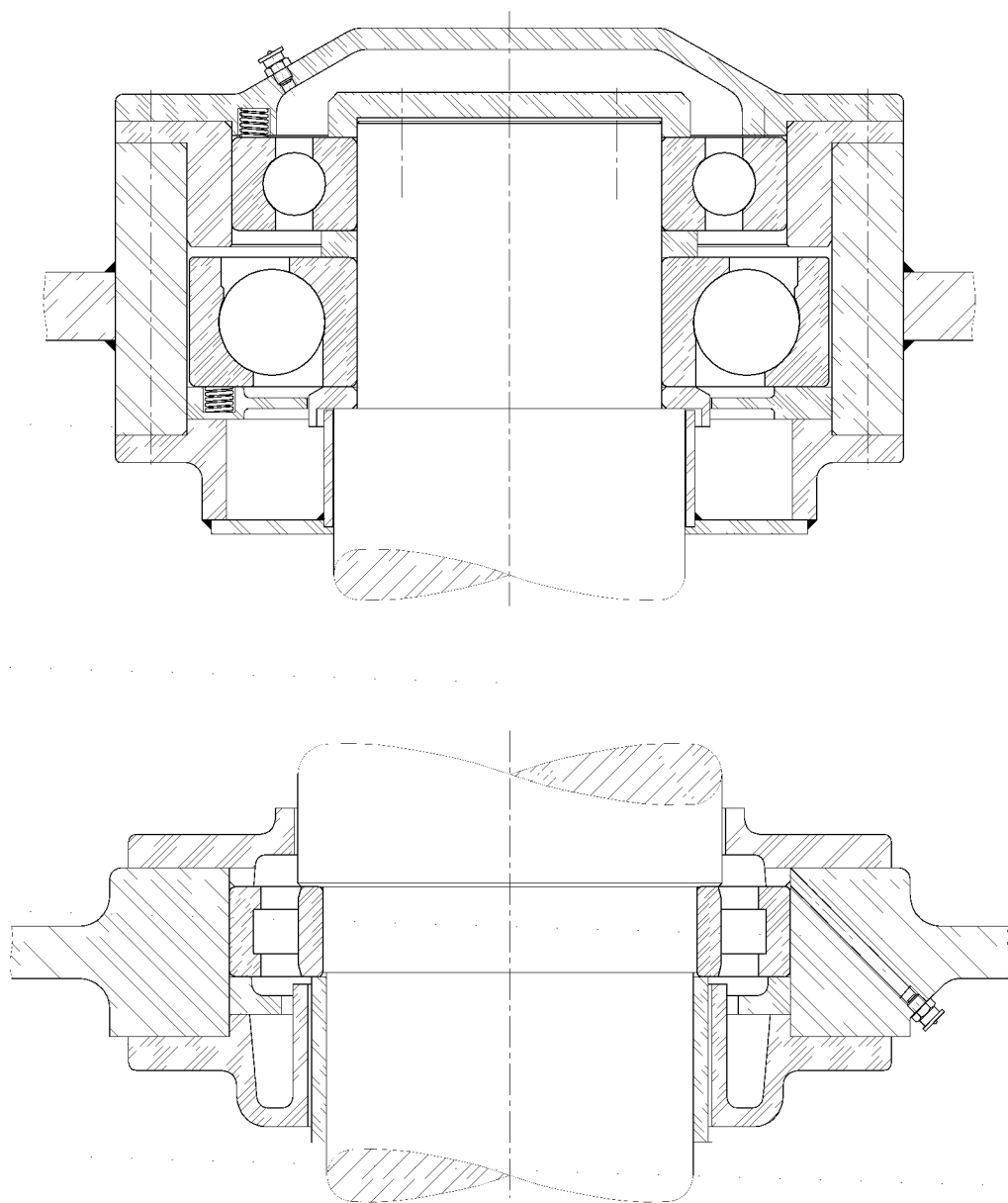
图 1-7 立式泵电动机转子轴承配置
