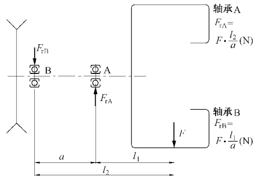
图 1-5 滚筒驱动示意图
