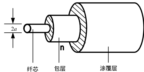
图 1-1 光纤结构图
