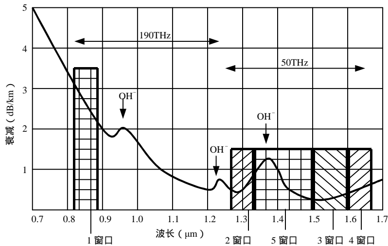
图 1-5 石英玻璃光纤的衰减
