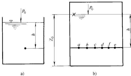
图(页) 液体内的压强和等压面
