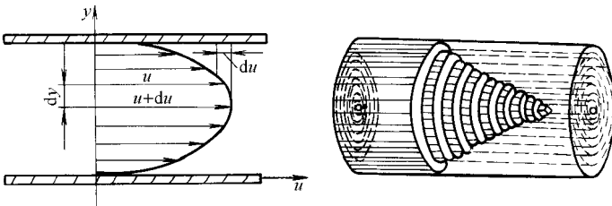
图 用 管内流速分布
