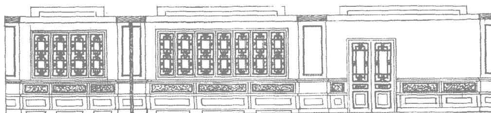
南立面图 1:50
