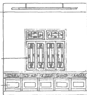
北立面 1:50
