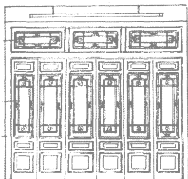
西立面 1:50
