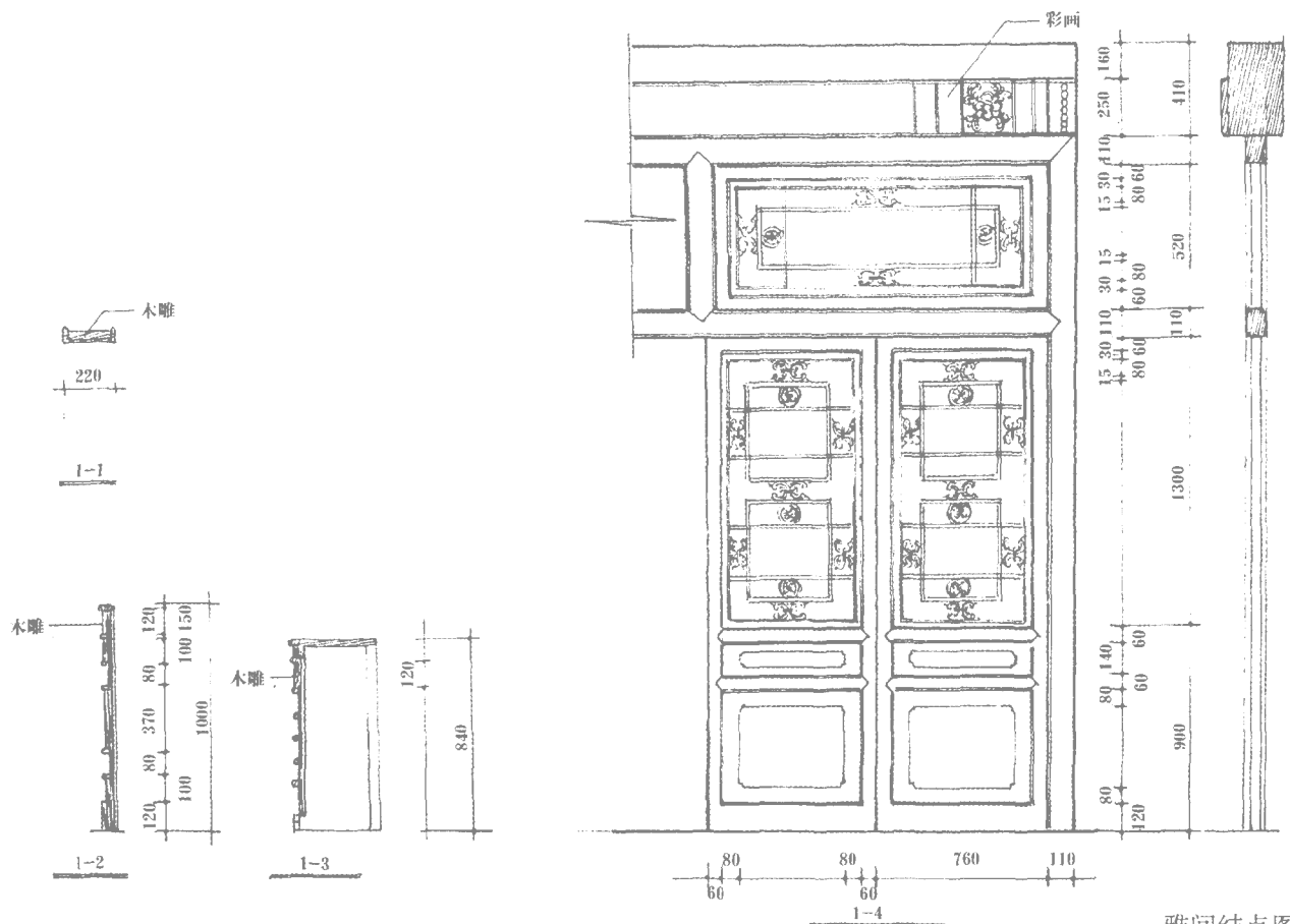
雅间结点图
