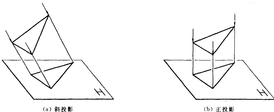
图 1-2-3 平行投影
