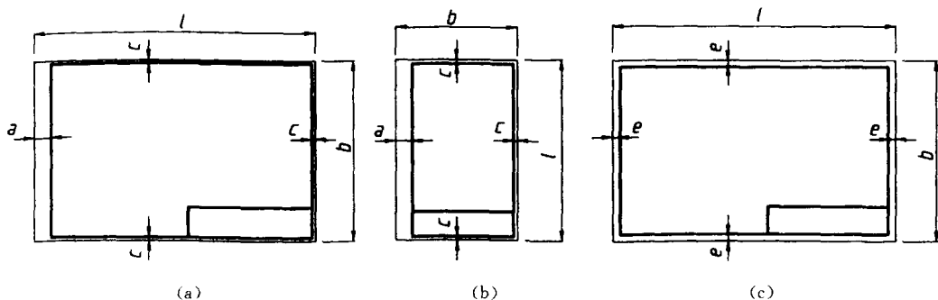
图 2-1-1 图幅和图框格式
