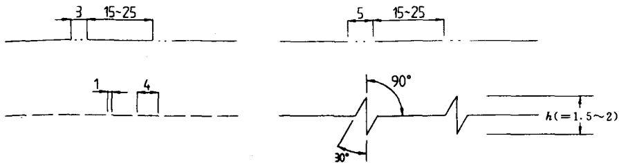
图 2-1-2 虚线、点划线和折断线的画法示例
