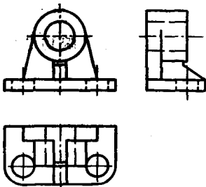
图 1-3-4 机件的正投影图
