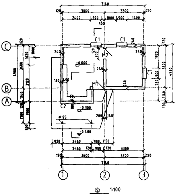
图 1-3-3 房屋的正投影图
