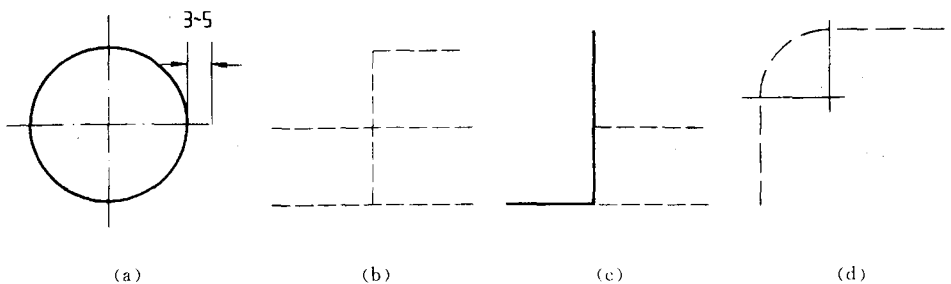
图 2-1-3 点划线和虚线的交接
