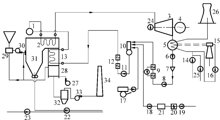
图 1-1 热力发电厂生产过程示意简图
