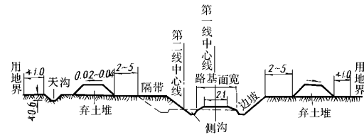
图 1—1—2 土质路堑标准横断面（单位：m）
