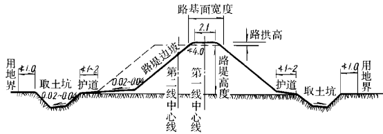
图 1—1—1 土质路堤标准横断面（单位：m）
