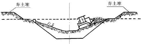
图 1—1—9 横向弃土开挖路堑
