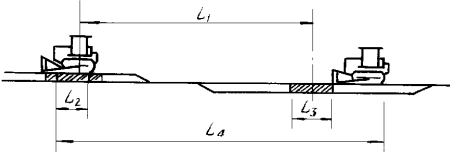
图 1—1—8 实际水平运距 L_1 ——定额水平运距； L_2 ——散土长度； L_3 ——切土长度； L_4 ——实际水平运距。
