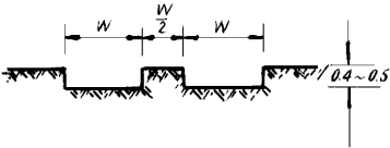
图 1—1—1 拉槽推土（单位：m） W——推土机刀片宽度。
