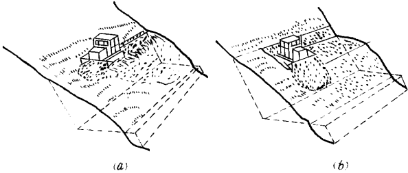
图 1—1—10 傍坡半路堑开挖 (a) 横推法；(b) 顺推法。
