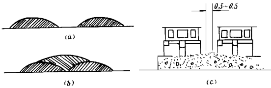
图 1—1—3 多刀推土填筑路堤（单位：m） (a) 四刀推土；(b) 六刀推土。L——推土距离。
