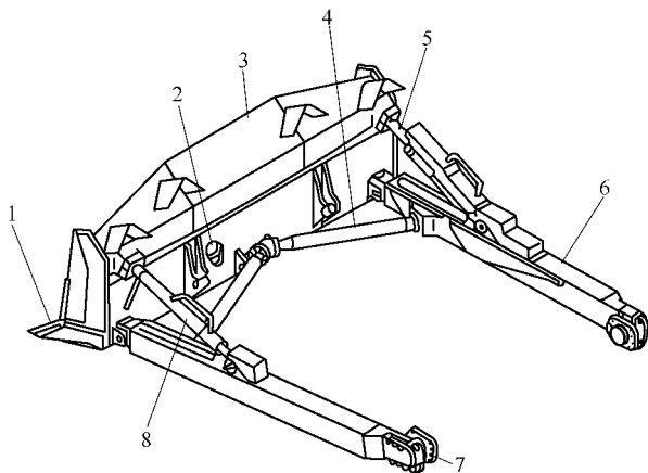
图 愿 愿 固定式推土装置
