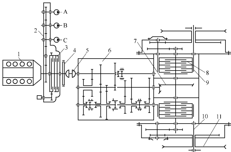
图 1 缘推土机的机械式传动布置简图
