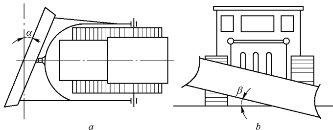
图 2-15 回转式铲刀安装示意图
