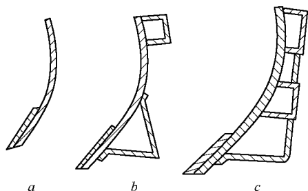
图 员圆 推土板断面结构形式 葬—开式；遭—半开式；糴—闭式
