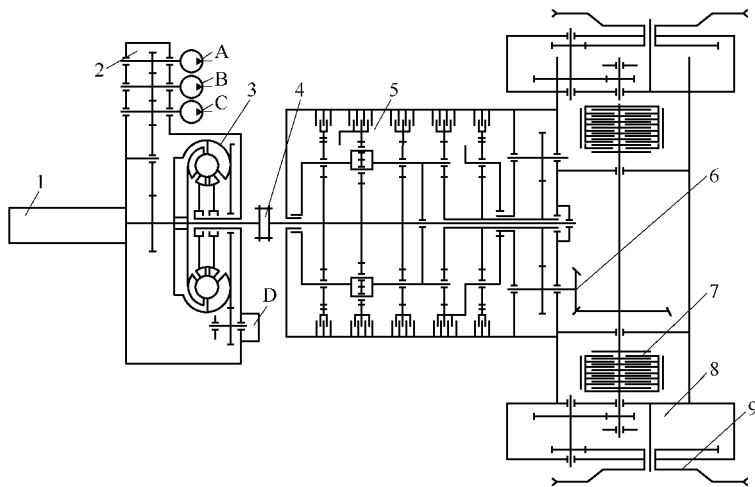
图 2 缘推土机液力机械式传动系统布置简图
