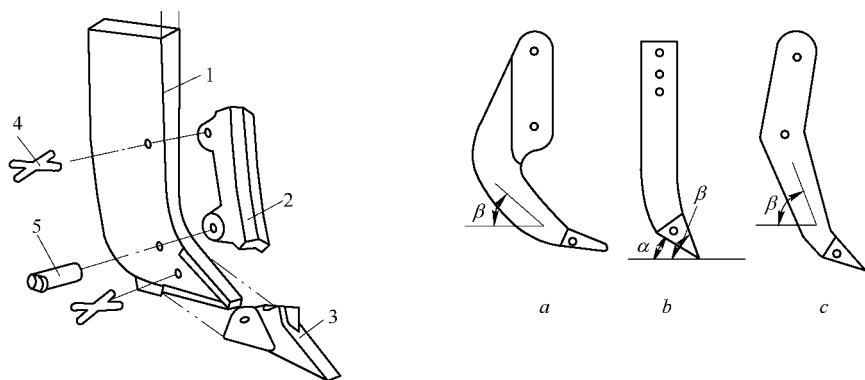
图 2 松土齿的构造
