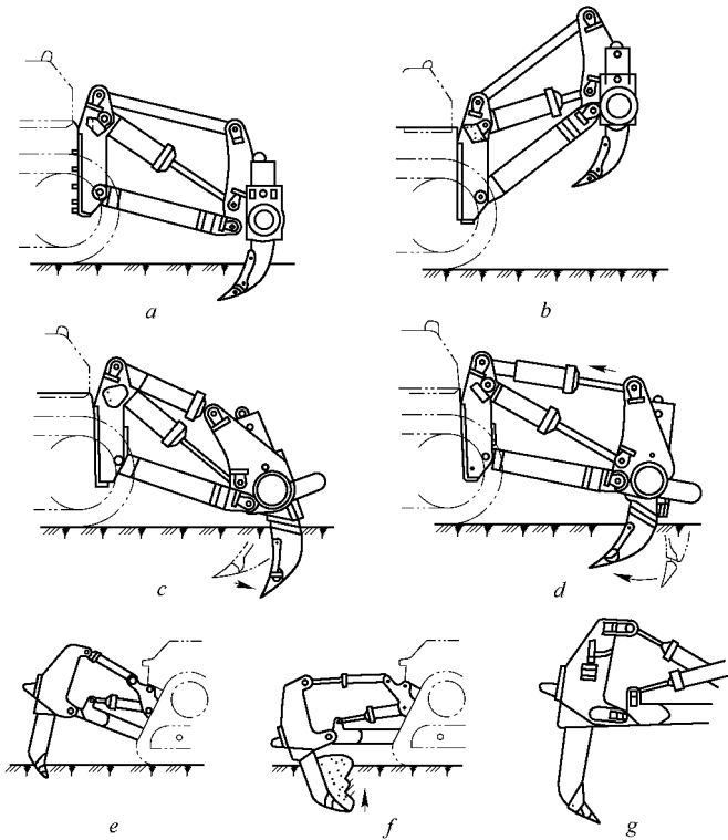
图 1-10 现代松土器的典型结构
