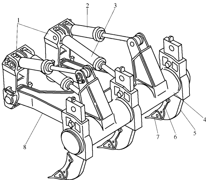
图 1 三齿松土器
