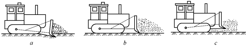
图 员圆 摇摇直铲式推土机的作业过程 葬—铲土作业；遭—运土作业；才—卸土作业
