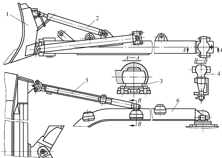
图 愿 愿 回转式推土装置
