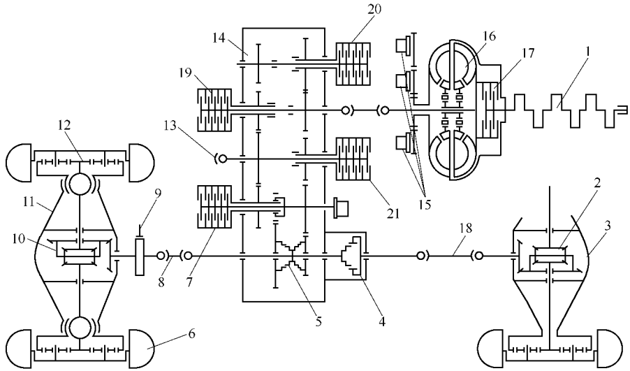
图 1-1 履带推土机的传动系统布置简图
