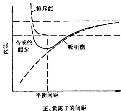
图2-1 从能量的观点分析离子键的形成
