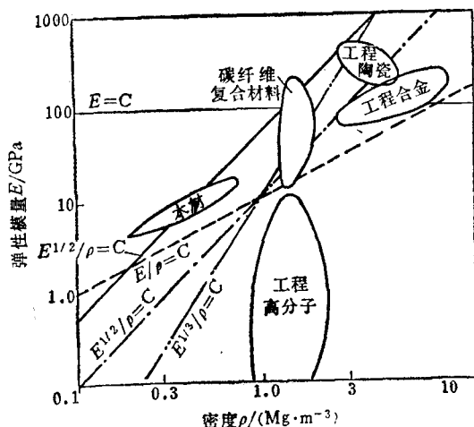
图1-1 材料的弹性模量—密度图
