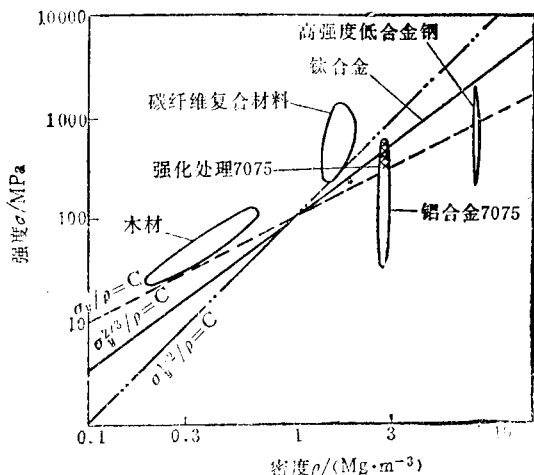
图1-3 材料屈服强度—密度图
