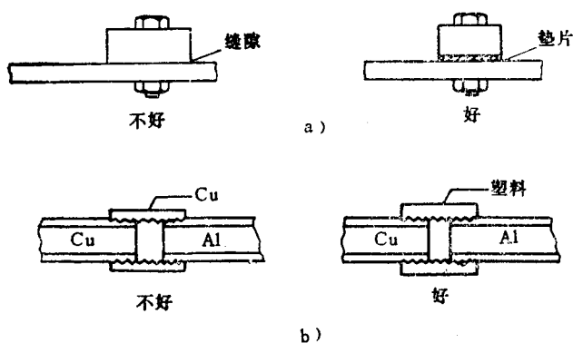
图1-4 防止缝隙腐蚀和电化学腐蚀
