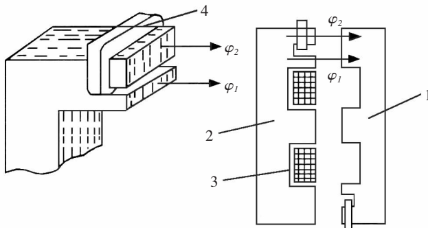
图 员原员 交流电磁铁的短路环 员原员 交流电磁铁的短路环 员原员 交流电磁铁的短路环
