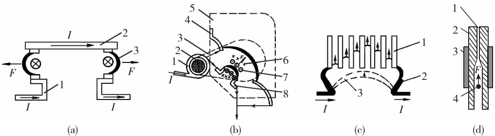
图 5-10 灭弧措施
