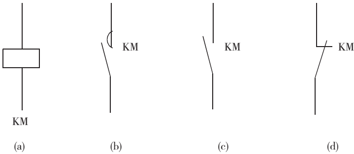
图 1-16 接触器的图形和文字符号
