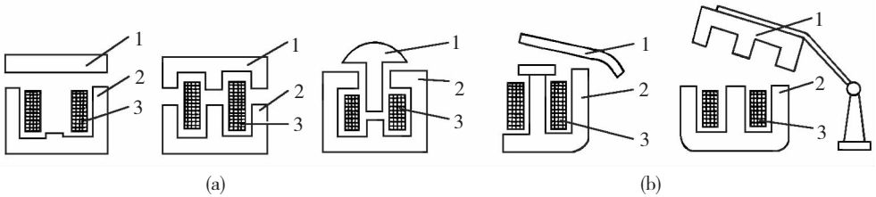
图 员原园 摇动式和拍合式电磁机构 (a) 摇动式电磁机构 (b) 拍合式电磁机构 员原园 摇动式电磁机构摇 (b) 拍合式电磁机构 员原园 摇动式电磁机构摇 (b) 拍合式电磁机构
