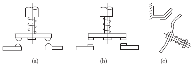
图 1-10 触头的结构形式
