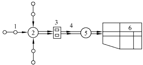
图 1-2 地下水源的给水系统
