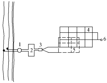
图 员猿源 分压给水系统
