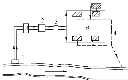
图 员京愿 循序给水系统 员—取水构筑物 圆—冷却塔; 猿—泵站 源—排水系统;粤—车间
