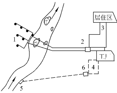
图 员猿猿 分质给水系统
