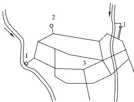
图 1-15 多水源给水系统 1—水厂 2—水塔 3—管网
