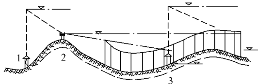
图 1-17 分区给水系统 1—低区供水泵站 2—水塔 3—高区供水泵站
