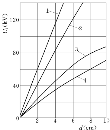
图 1-8 直流电压下间隙放电电压与间隙距离的关系曲线
