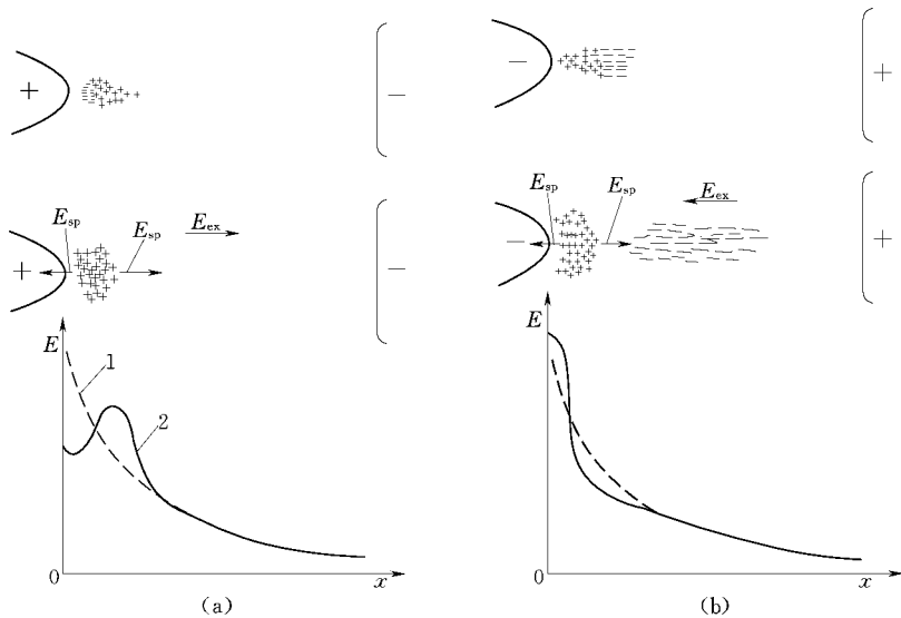
图 1-7 棒板间隙起始放电示意图
