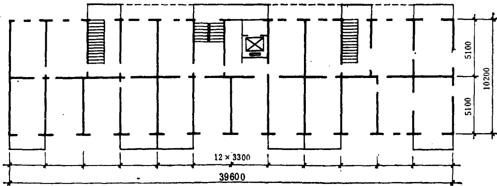
(a) 高层板式楼平面
