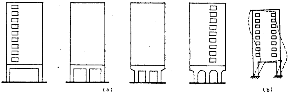
图1-7 框支剪力墙
