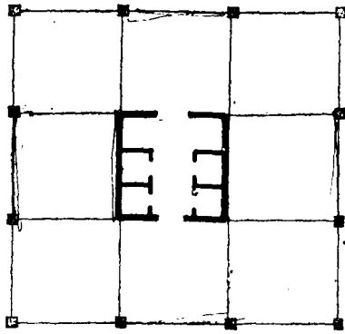
图1-11 框架-筒体结构的典型布置
