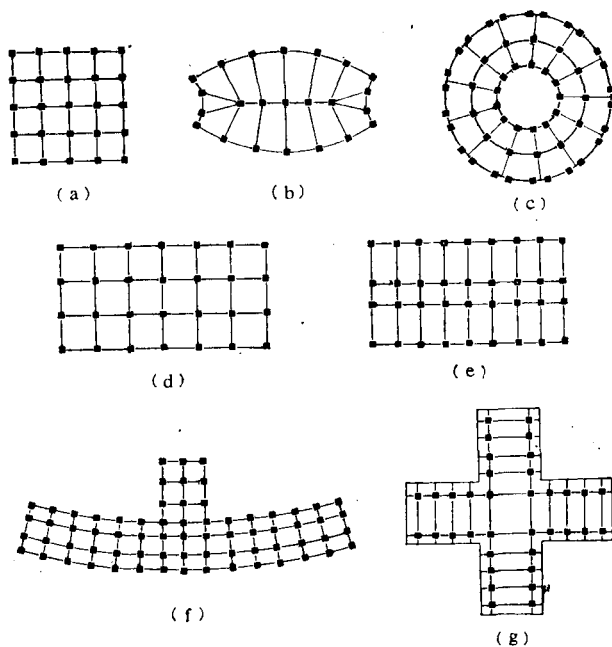
图1-3 框架柱网布置举例
