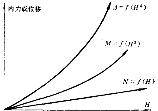
图1-1 结构内力、位移与高度的关系
