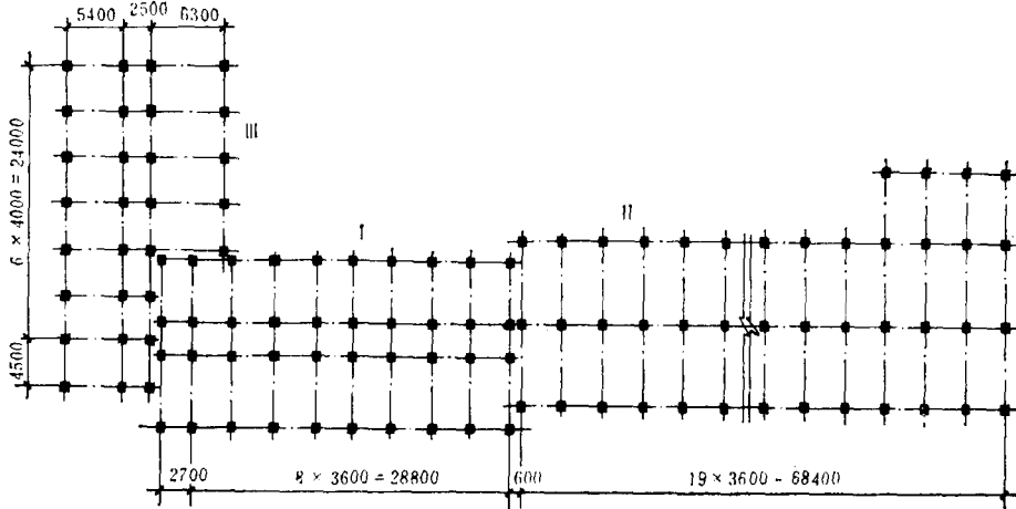
图1-4 北京民航大楼框架柱网布置
