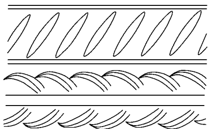
图 1-1 月牙肋钢筋外形
