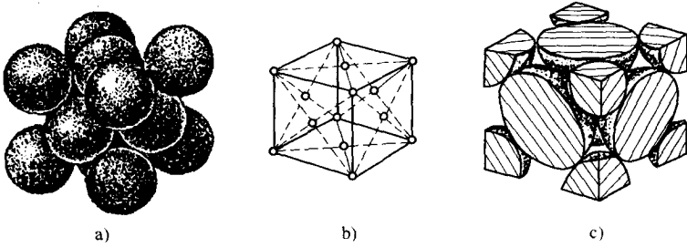
图 1-4 面心立方晶胞 a)刚球模型;b)质点模型;c)晶胞原子数
