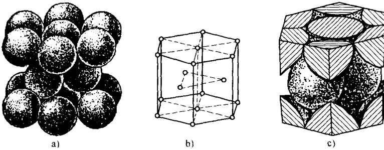
图 1-5 密排六方晶胞 a)刚球模型;b)质点模型;c)晶胞原子数
