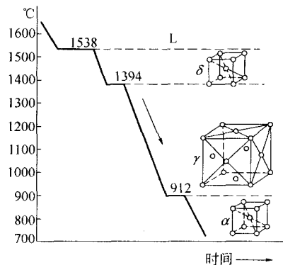
图 1-7 纯铁的冷却曲线
