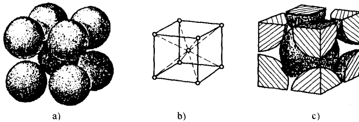
图 1-3 体心立方晶胞 a) 刚球模型; b) 质点模型; c) 晶胞原子数
