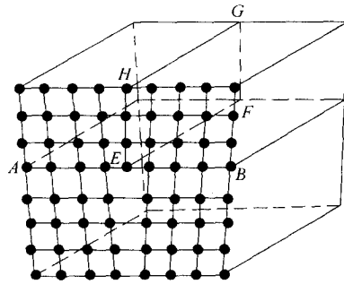
图 1-12 刃型位错示意图
