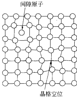
图 1-11 晶格点缺陷
