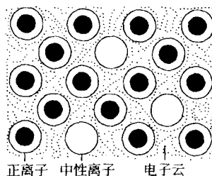
图 1-1 金属键模型
