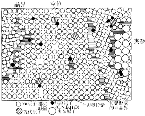
图 1-10 实际金属晶体的结构
