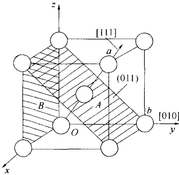
图 1-6 晶面和晶向
