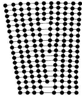
图 1-13 亚晶界图
