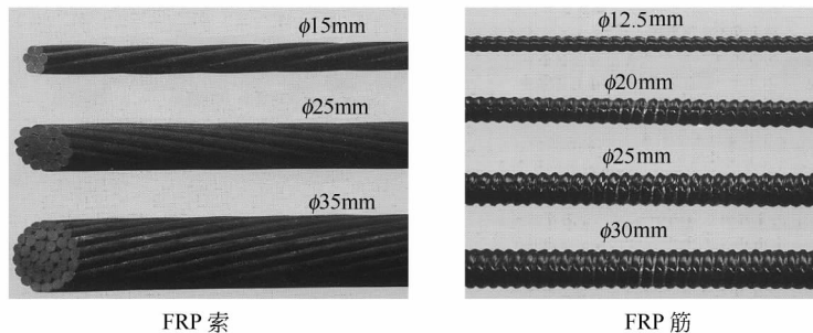
图 1-3 FRP 索与 FRP 筋
