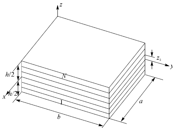
图 2-1 摇 层板几何图形
