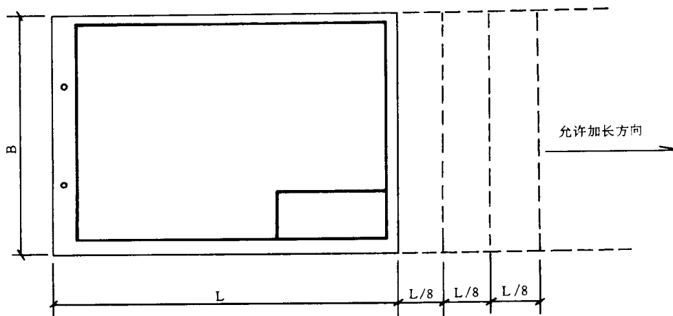
图 1-22 制图图纸格式
