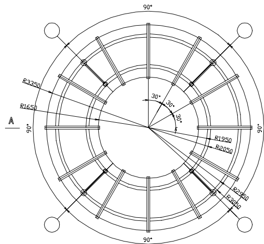
景亭平面图
