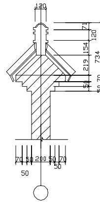
山墙脊剖面图
