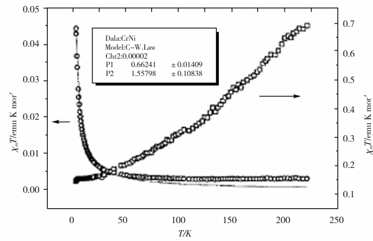
图 2 配合物 B 的 \chi_m \sim T 和 \chi_m T \sim T 曲线
