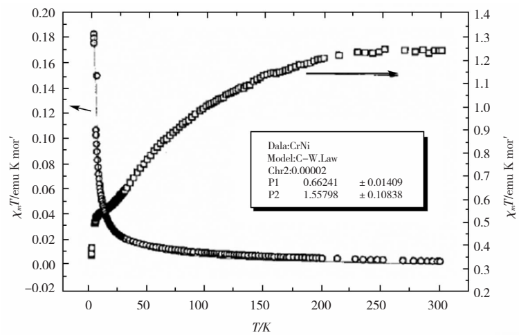
图 1 配合物 A 的 \chi_m \sim T 和 \chi_m T \sim T 曲线
