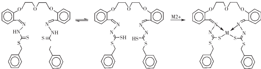
图 1 H_2L 两种互变异构体及 ML 配位模式
