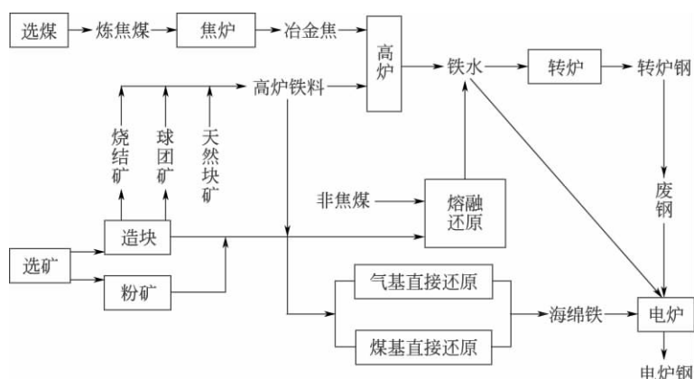
图 1-2 现代钢铁生产全流程解析
