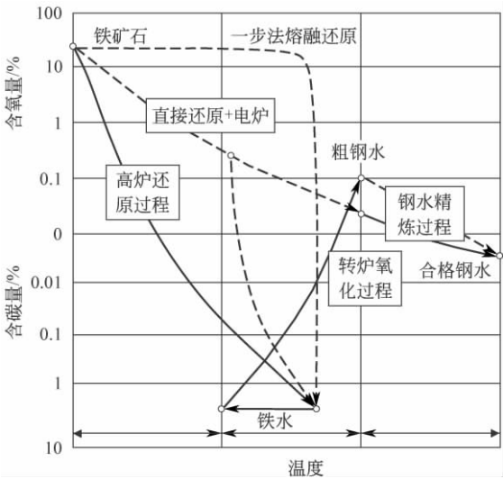
图 1-4 钢铁生产过程产品中含氧量、含碳量的变化示意
