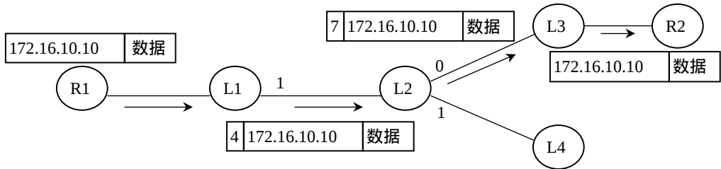
图 1.4 MPLS 系统示意图
