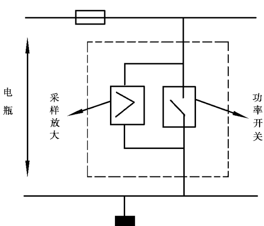
图 1-1-3 过压保护器示意图
