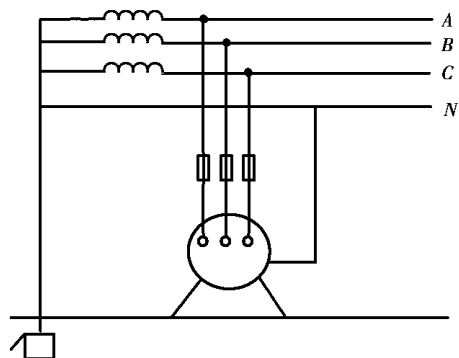
图 1-1-2 接零保护示意图
