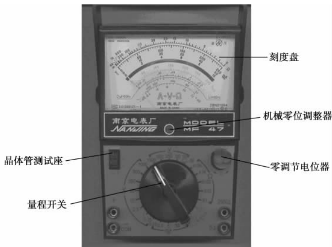
图 1-1 MF47 型指针式万用表面板
