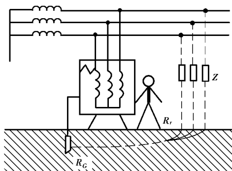
图 1-1-1 接地保护示意图
