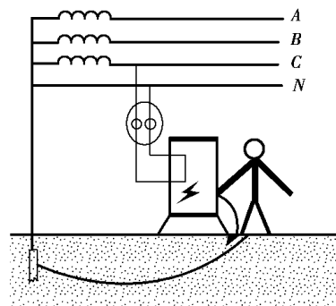
图 猿猿猿 单相触电示意图
