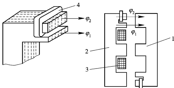
1—衔铁；2—铁心；3—线圈；4—短路环
