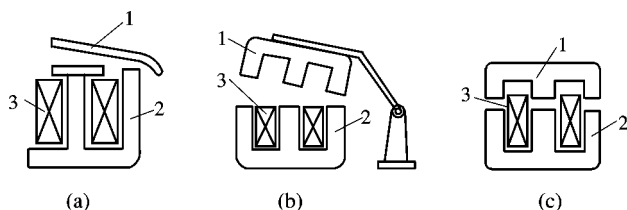
1—衔铁；2—铁心；3—吸引线圈
