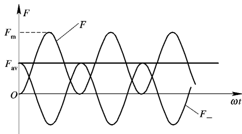
图 1-2 交流电磁铁吸力变化情况
