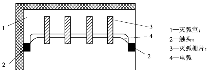
图 1-7 金属栅片灭弧示意图
