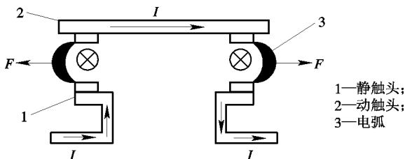
图 1-5 双断点触头的电动力灭弧
