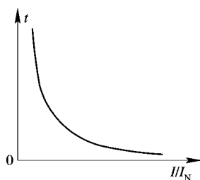
图 1-8 熔断器的安秒特性
