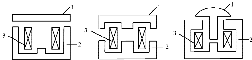
图 1-10 直动式电磁机构 1—衔铁；2—铁心；3—吸引线圈
