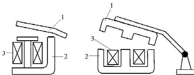
图 1-11 拍合式电磁机构 1—衔铁；2—铁心；3—吸引线圈
