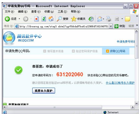
图 7-12 申请成功
