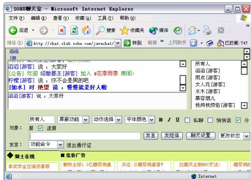
图 7-4 进入聊天室
