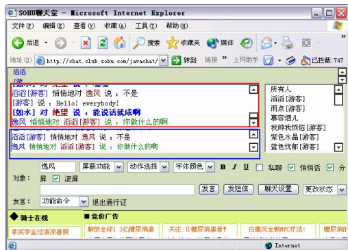
图 7-5 聊天室界面
