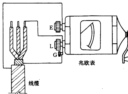
图 1-2-3 需屏蔽测试时兆欧表接线
