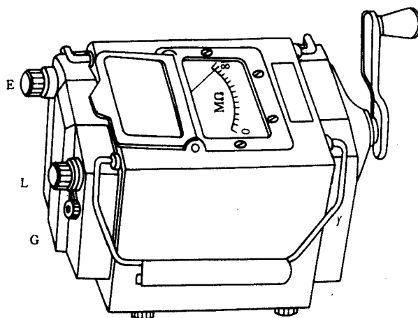
图 1-2-1 兆欧表外形
