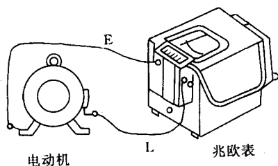
图 1-2-2 兆欧表一般接线
