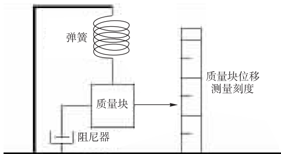
图 5-1 惯性地震计工作原理示意图
