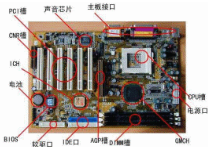
图 1-1 主板结构图
