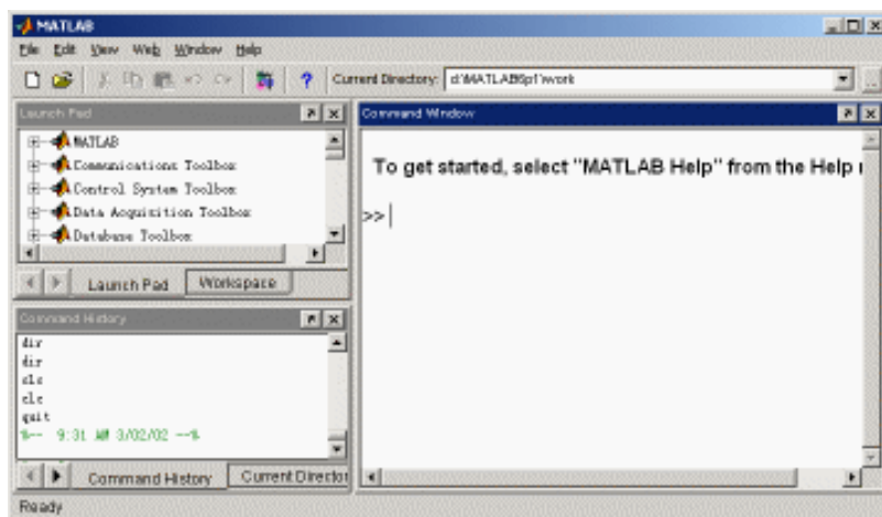
图 1.5 MATLAB 界面
