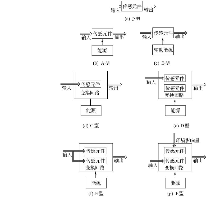
图 1-1 传感器组成框图
