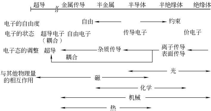
图 1-3 物质中电子自由度及其调整与化学、物力的相互作用
