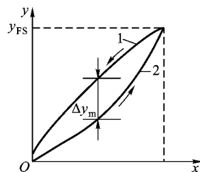
图 1-4 迟滞特性图
