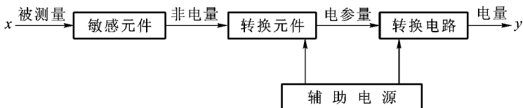
图 1-1 传感器组成框图
