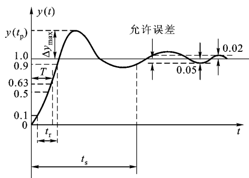
图 1-6 阶跃响应曲线图
