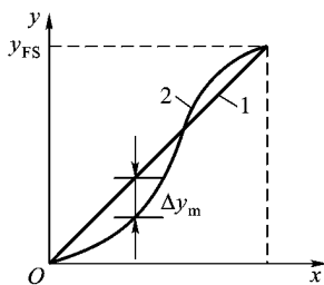
图 1-3 特性曲线与线性度关系曲线
