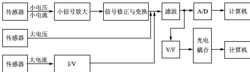
图 2-1-4 大信号输出传感器的使用
