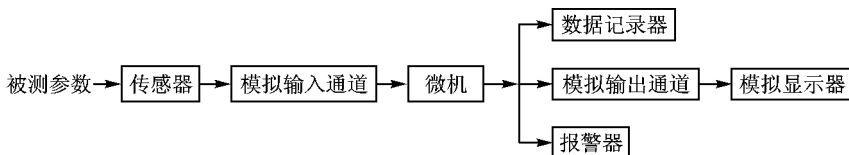
图 1-3-1 微机化检测系统框图
