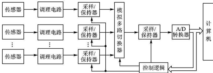
(b) 多路同步采集分时输入结构
