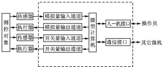
图 1-3-3 微机的测控系统典型结构
