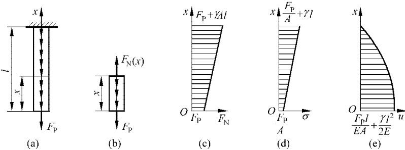
图 员源 考虑自重时的杆件应力、变形计算
