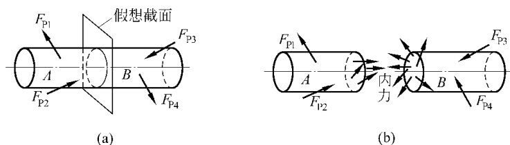
图 1-1 轴拉压杆件内力与截面法
