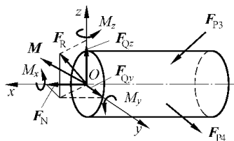
图 1-2 轴拉压杆件横截面上的内力分量
