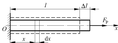
图 1-10 轴向载荷作用下杆件的纵向变形和横向变形
