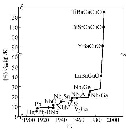
图 展示了超导材料的进展
