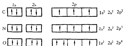
图 1 2 碳、氮、氧原子的电子层排布
