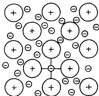
图 1 4 金属键示意图
