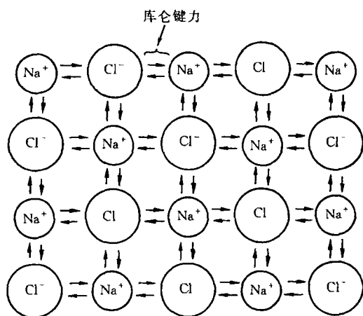
图 1 5 NaCl 离子键的示意图
