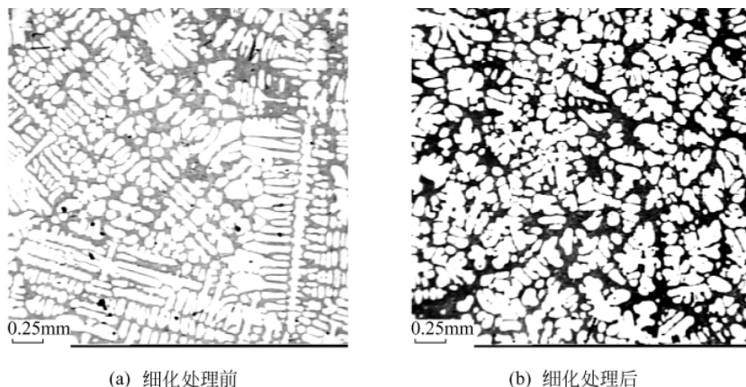
图 1-10 铝硅合金细化处理前后的显微组织
