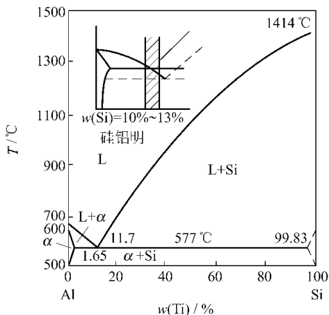
图 1-10 铝硅二元相图
