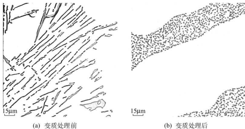
图 员源 铝硅合金变质处理前后的显微组织
