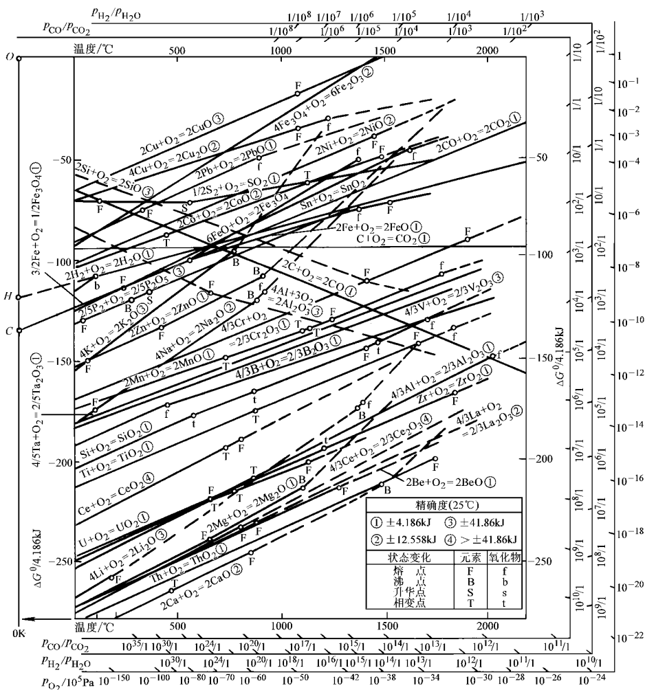
图 10-1 一些氧化物的 \Delta G^\circ 图
