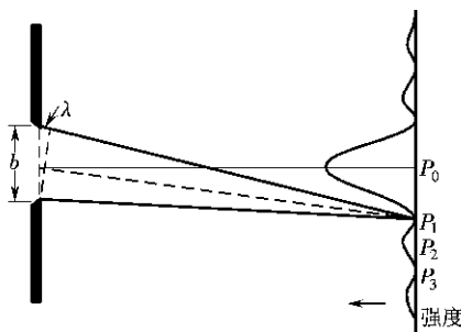
图 1.2-1 光波衍射示意图
