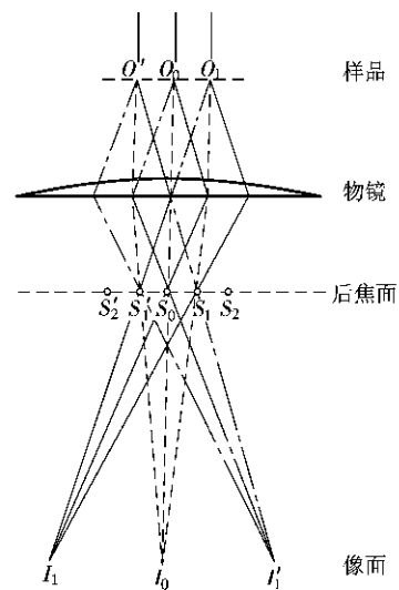
图 4-2 光线经过周期性结构的物体时的衍射现象
