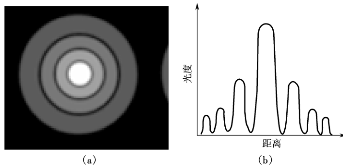
图 4-1 由于衍射效应而形成的埃利斑 (a) 由斑点光源衍射形成的埃利斑 (b) 光强分布图
