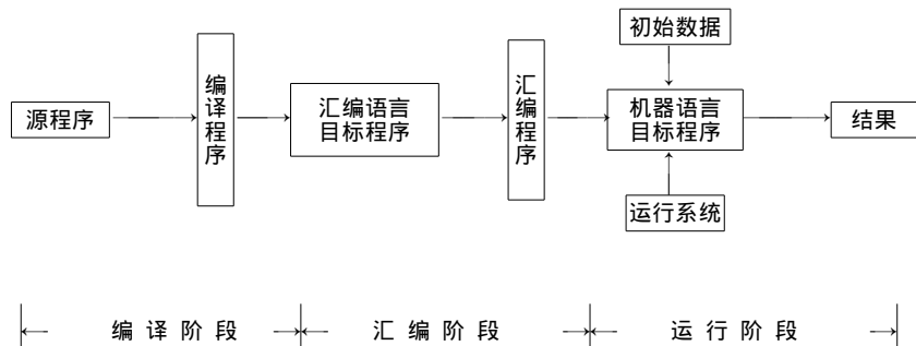
图 1.1 源程序的编译、汇编和运行阶段
