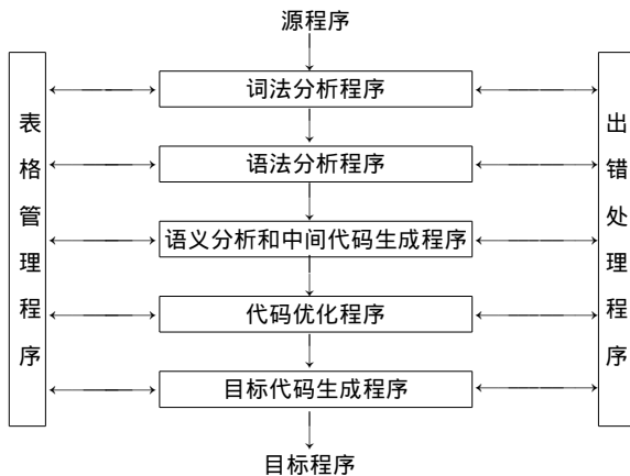
图源缘 编译程序结构框图
